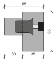
Einbaugeschäuse von der Seite
