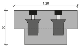
Einbaugeschäuse von oben
